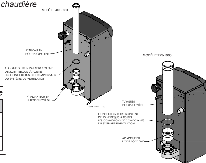
Figure 3-5 Ventilation en Polypropylène à proximité de la chaudière
