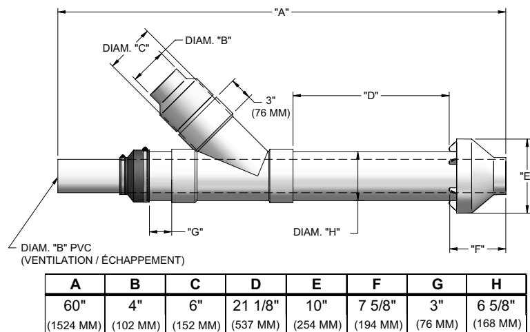
Figure 4-9 Schéma des dimensions de ventilation concentrique - Modèles 400 - 600
