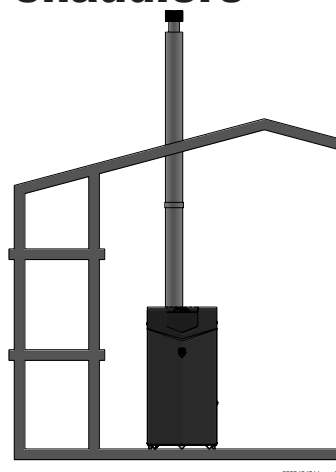
Figure 1-4_Air de combustion par conduites
