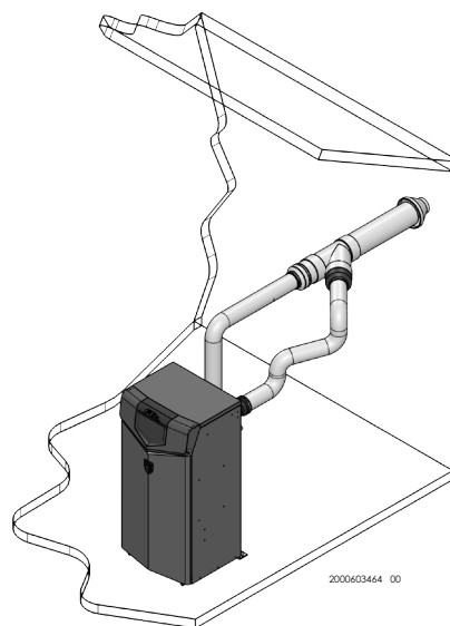
Murale concentrique en PVC/CPVC Modèles 400 - 600 uniquement Voir page 28 pour d'autres détails
