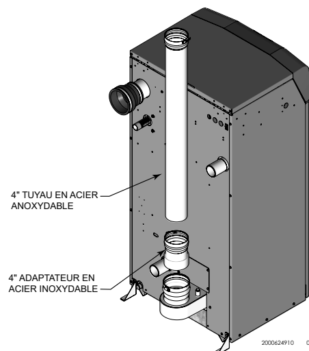
Figure 3-7 Près de la ventilation en acier inoxydable du chaudière modèles 725 - 1000
