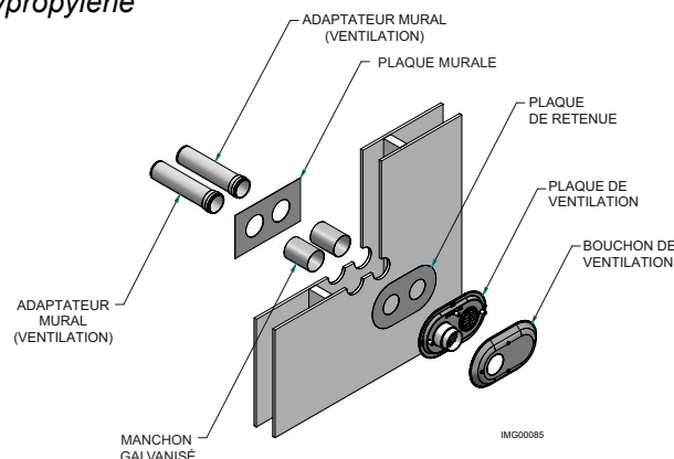
Figure 4-5C Ensemble de terminaison murale en polypropylène
