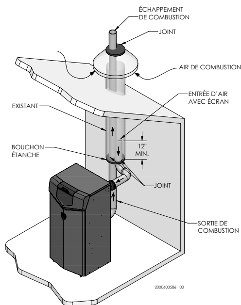
Figure 5-8 Exemple 1 de ventilation concentrique
